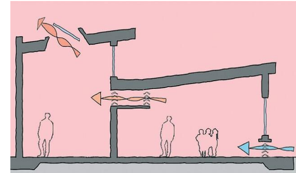
Ventilazione naturale
